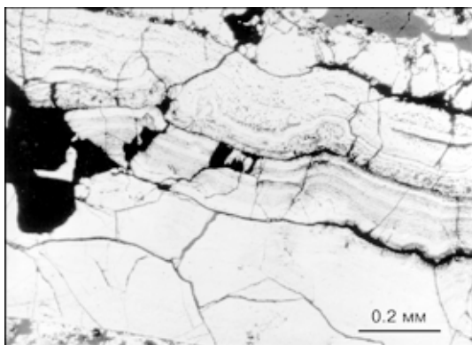
Рис. 88. Марказит-пиритовое бактериальное обрастание вокруг трубки вестиментиферы. Состоит из трех частей: внутренней – массивной пористой, средней – ламинарной и верхней – фрамбоидальной. Отраженный свет. Месторождение Яман-Касы.
