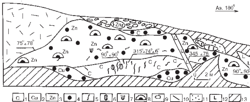
Рис. 63. Строение холмообразной сульфидной постройки.
