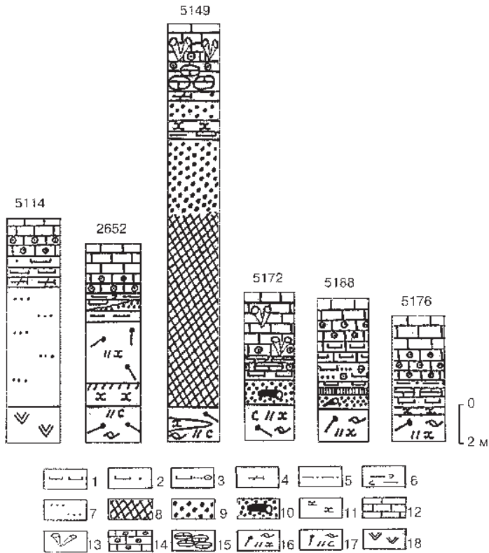
Рис. 30. Литологические колонки второго (госсанитового) горизонта кремнисто-железистых пород по субширотному разрезу.
