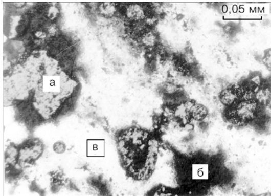
Рис. 45. Замещение пирита (а) гематитом (б) в кварц-хлоритовом агрегате (в).
