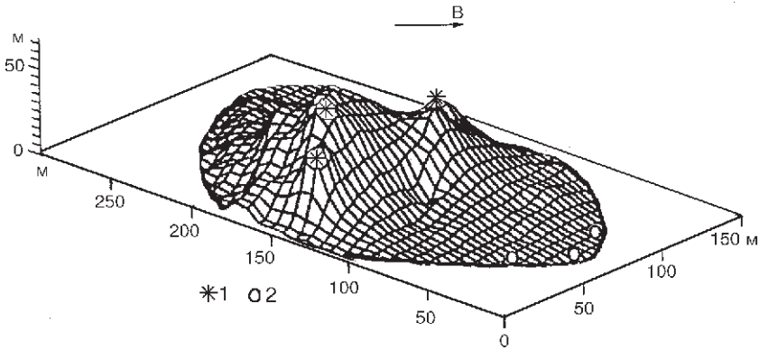
Рис. 67. Локализация оруденелой фауны в сульфидной гидротермальной постройке месторождения Яман-Касы.
