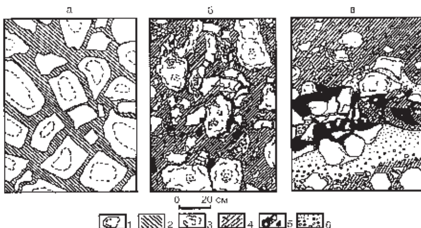
Рис. 40. Обломочные руды кровли сульфидной залежи месторождения Яман-Касы.
