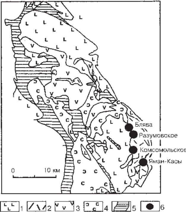
Рис. 2. Схема размещения колчеданных месторождений в Медногорском районе.
