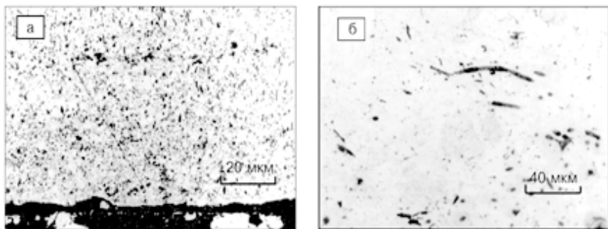
Рис. 89. Нижняя часть пирит-марказитового бактериального обрастания (см. рис. 88). а – общий вид: видны псевдоморфозы кварца (черное) по бактериоморфным нитям. Отраженный свет.
